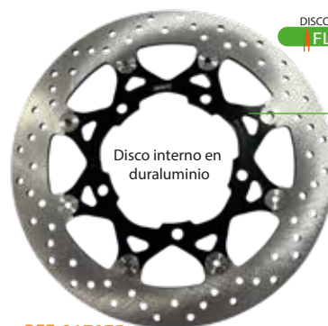
REF. 217075 DISCO DE FRENO FLOTANTE DE SUZUKI VSTROM650 CLASSIC - 650 ABS - GSR600 MV - GSF BANDIT 650 MV- GSR750- GSX S750- GSF BANDIT 1250
