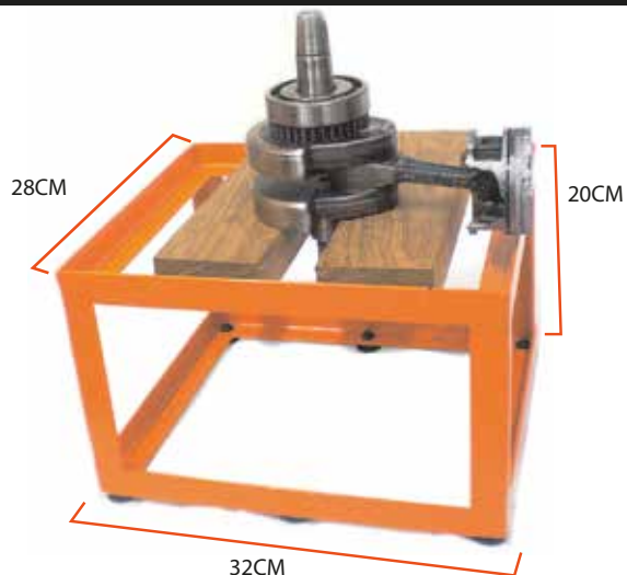
REF: 207110 SOPORTE ARMA-MOTOR, ANTIDEZLIZANTE
